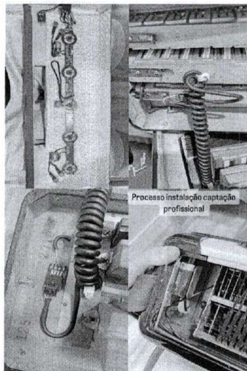
Figura 4- Instalação de Captação em Acordeon
